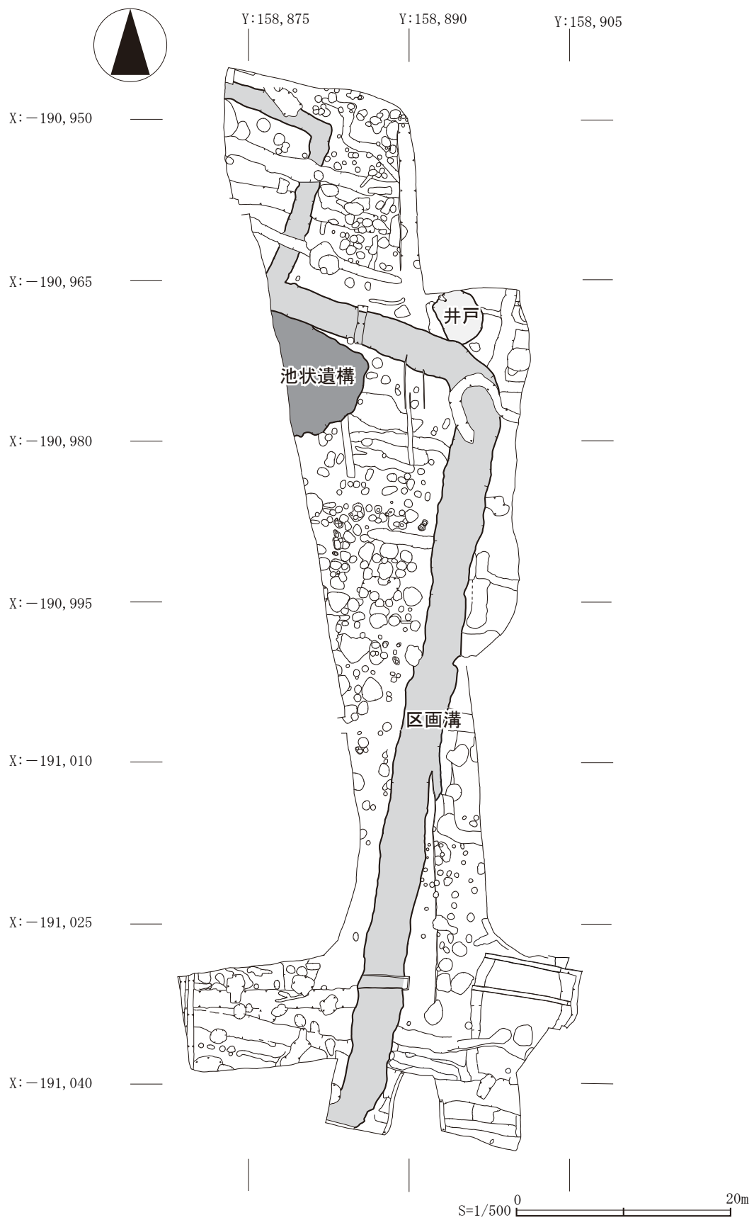
第4図 1区 遺構平面図
