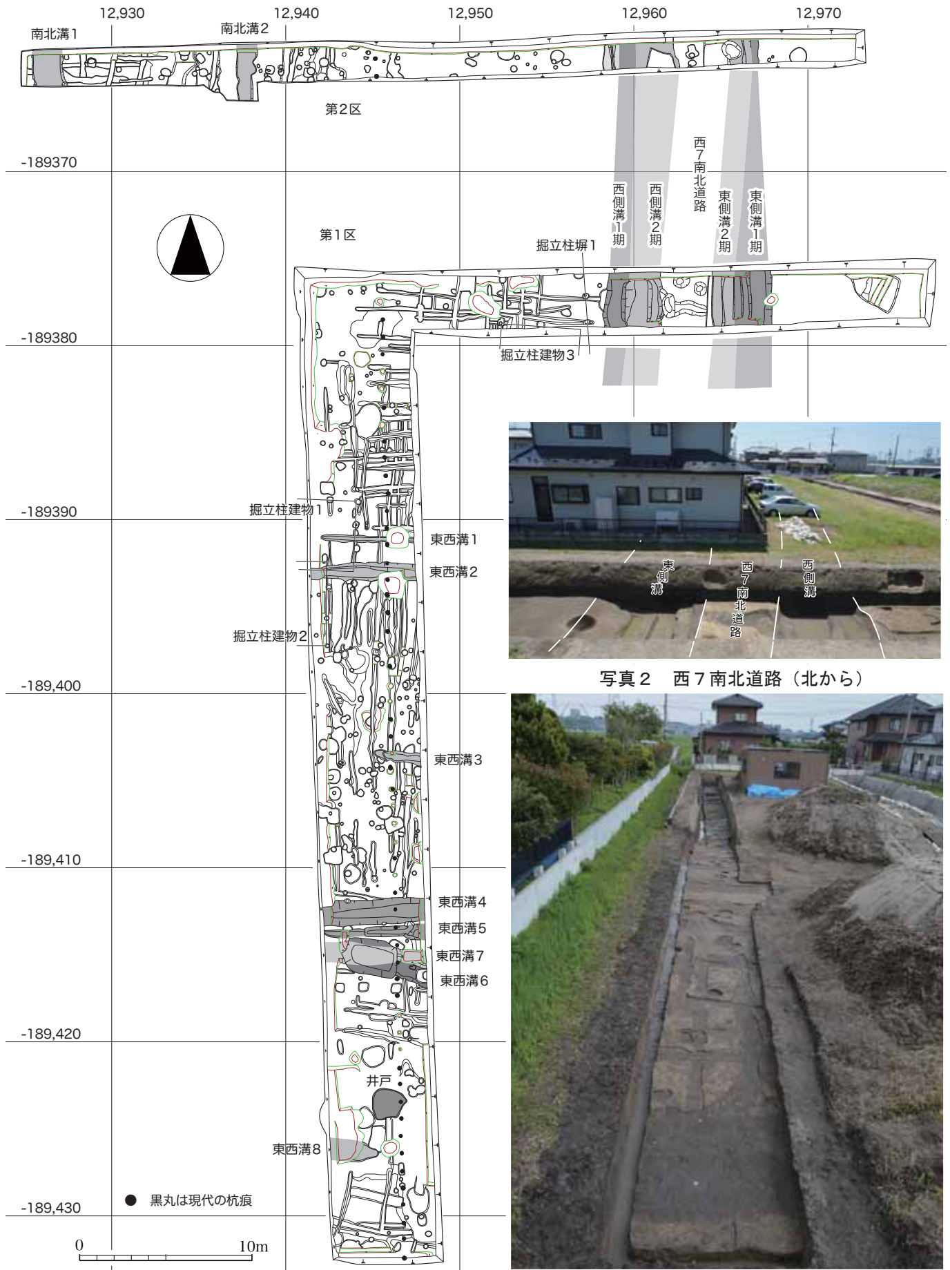
第2図 調査区平面図 (1/300)
