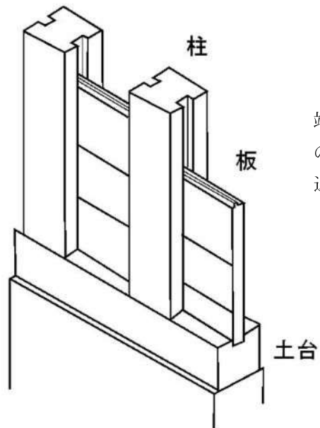
板倉の構造
