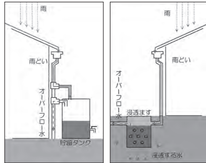
雨水貯留タンクの設置例
