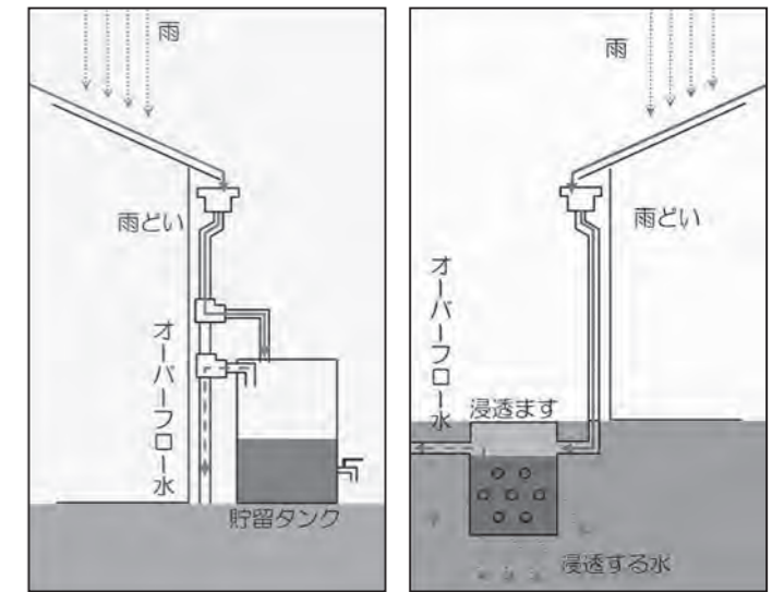
雨水貯留タンクの設置例
