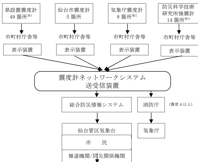
【宮城県震度情報ネットワークシステム概要図】
